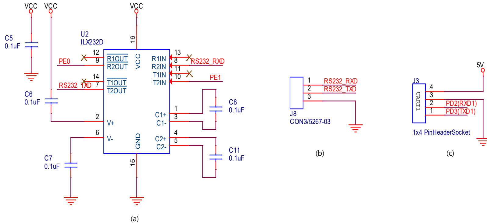
Figure 5. 회로도 트랜시버 IC MAX232(a), RS232통신 송수신 3P 몰렉스 커넥터(b), UART1 통신포트 4P 핀 헤더 소켓 커넥터(c)
